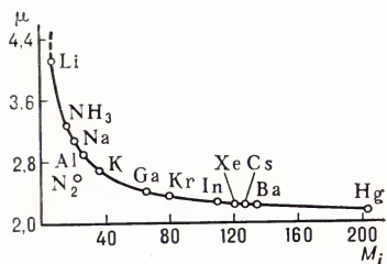
Рис. 2. Зависимость подвижности ионов \mu от их массы M_i .
